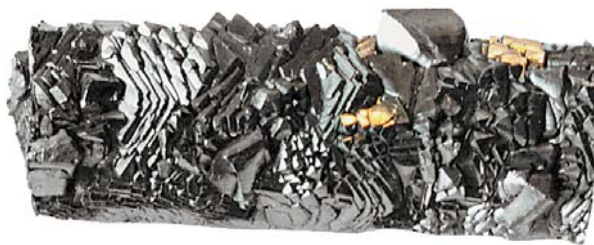
Кристалл титана, очищенного иодидным методом.
