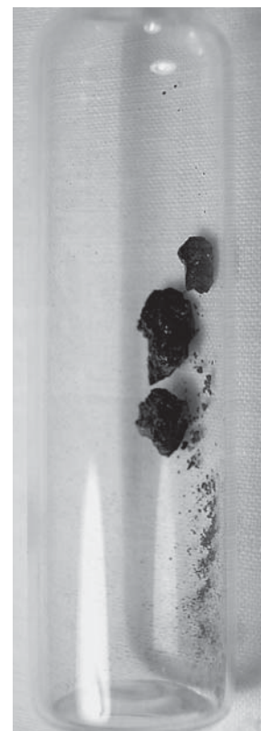
В этом образце уранового минерала содержатся ничтожные количества астата.
