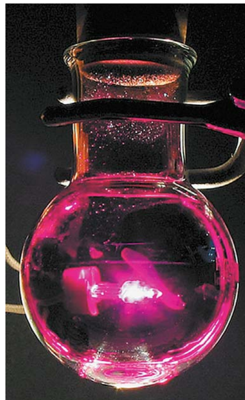
Пары иода имеют темно-фиолетовый цвет.
