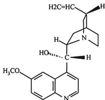
Хинин
