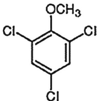
Трихлоранизол
