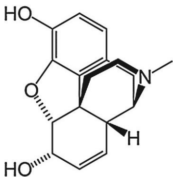
Морфин
