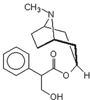
Атропин
