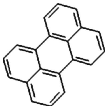
Перилен
