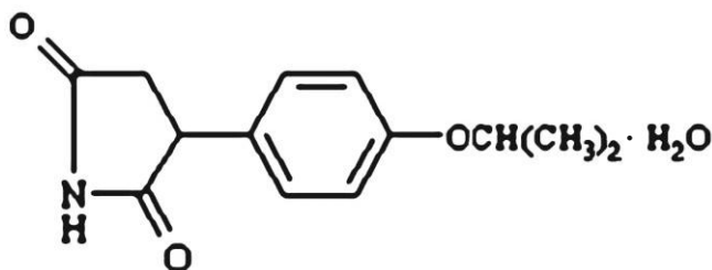
Пуфемид
