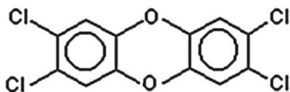
Формула 3,4,7,8-тетрахлордибензодиоксины
