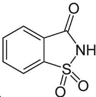
Сахарин
