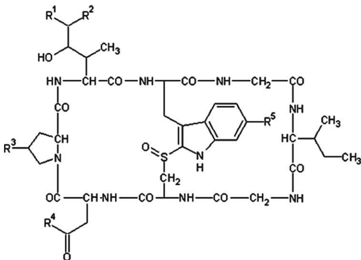
Аманитин
