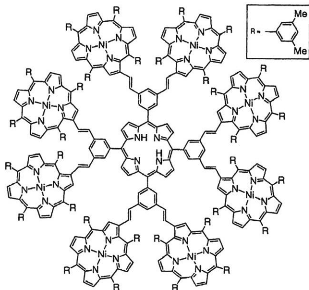
Структура 48
