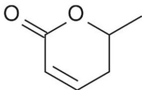
Лактон
