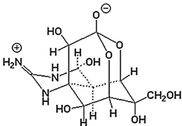
Тетродотоксин
