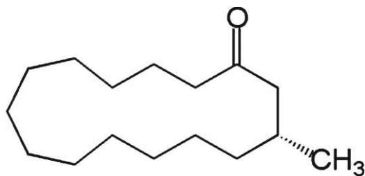
Мускон
