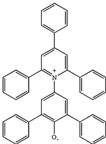
Структура 47
