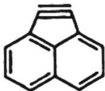
Аценафтин
