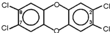
Диоксин
