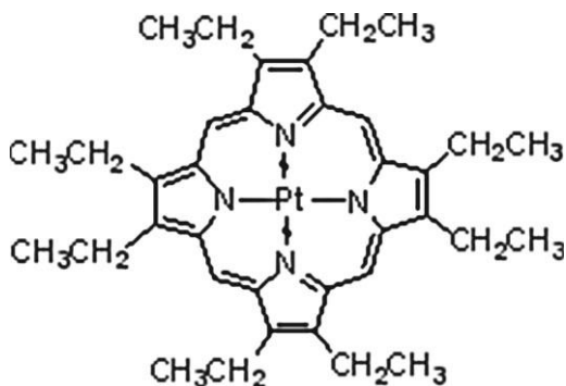
Октаэтилпорфирин (комплекс с платиной)
