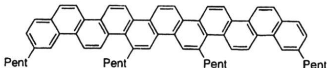
Структура 37
