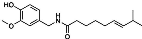
Капсаицин
