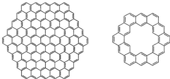
Структуры 38, 39
