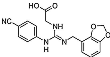
Лугдунам
