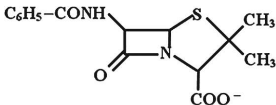
Бензидпенициллин
