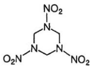
Структуры 23, 24, 25, 26
