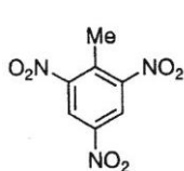
Структуры 23, 24, 25, 26
