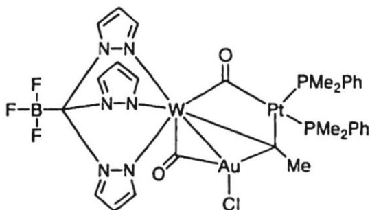
Структура 46
