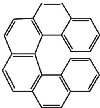
Гексагелицен
